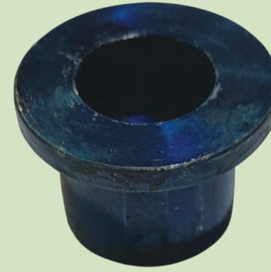
MS BUSH (OD 54 MM X ID 28 MM X 36 MM LONG)
